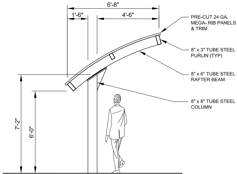
ELEVATION SCALE: 1/4" = 1'-0"
