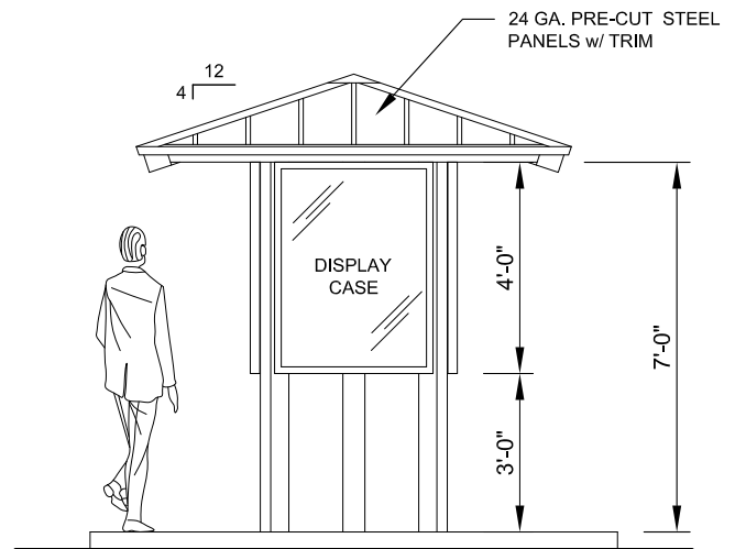
ELEVATION SCALE: 1/4" = 1'-0"
