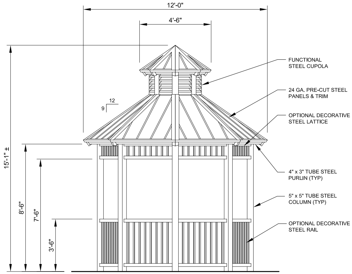
ELEVATION SCALE: 1/4" = 1'-0"
