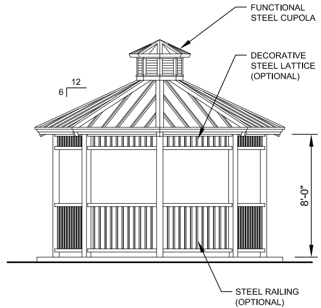
ELEVATION SCALE: NTS
