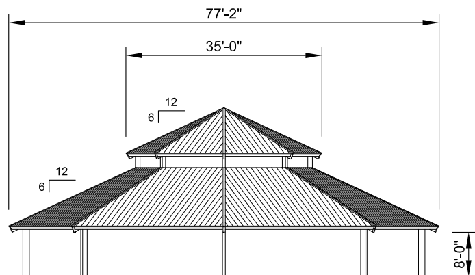
ELEVATION SCALE: NTS
