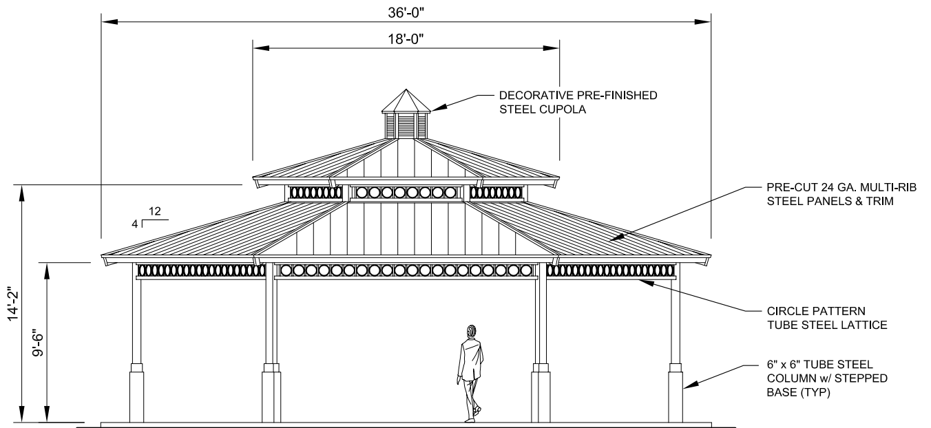
ELEVATION SCALE: NTS
