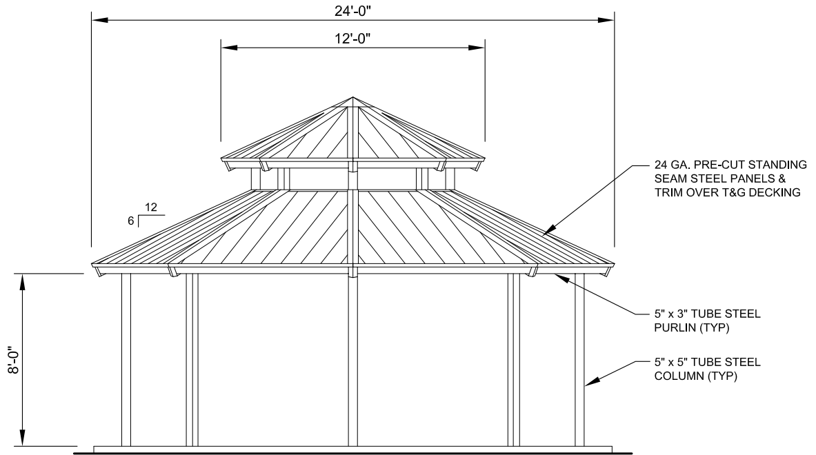
ELEVATION SCALE: NTS
