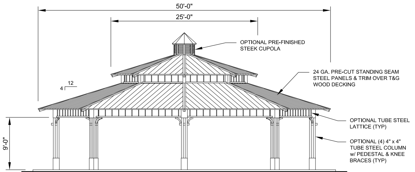
ELEVATION SCALE: NTS
